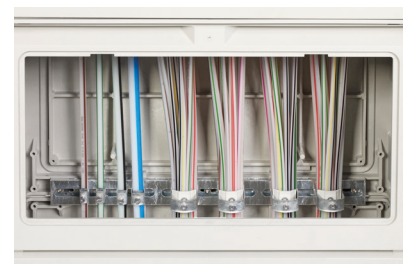
▲ Sockel mit geöffneter Klappe und montierten Mikrorohren
